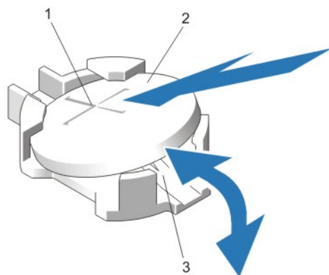
Ilustración 35. Sustitución de la batería del sistema
