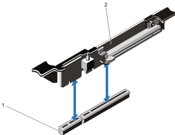
Ilustración 22. Extracción e instalación de la tarjeta vertical de expansión 3
