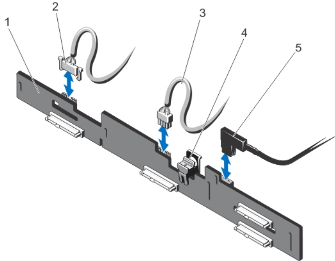
Ilustración 36. Extracción e instalación del plano posterior de la unidad de disco duro (x4) de 6,35 cm 2,5 (pulgadas)
