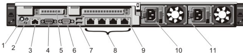
Ilustración 4. Características e indicadores del panel posterior
