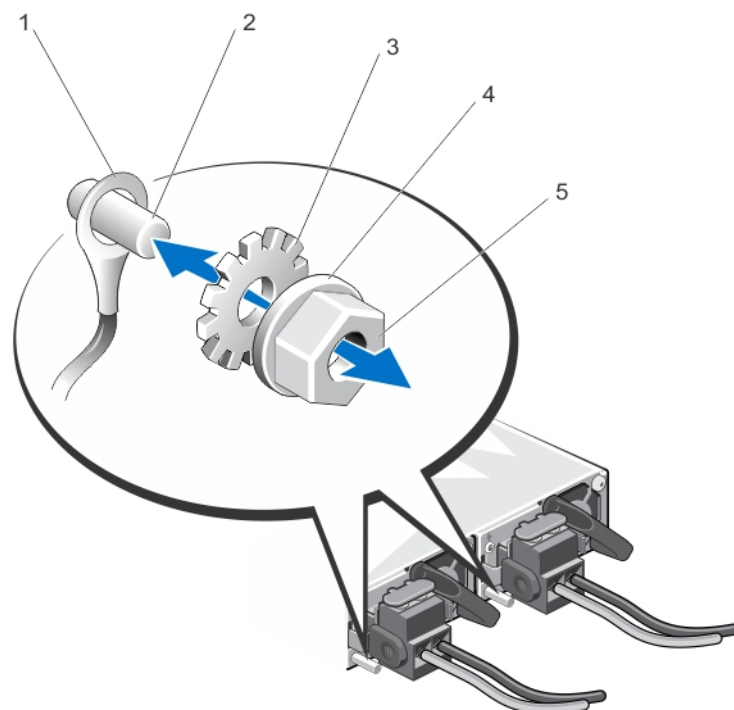
Ilustración 30. Ensamblaje y conexión del cable de toma a tierra de seguridad
