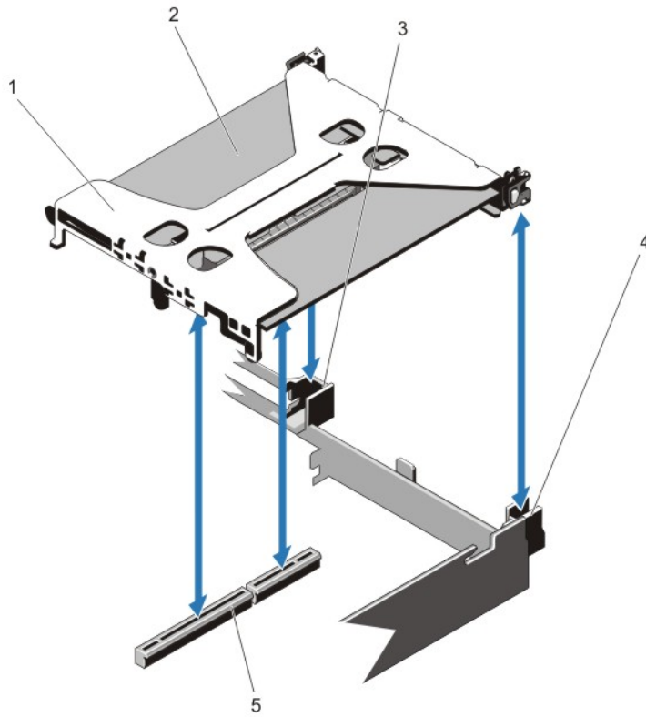
Ilustración 21. Extracción e instalación de la tarjeta vertical de expansión 1
