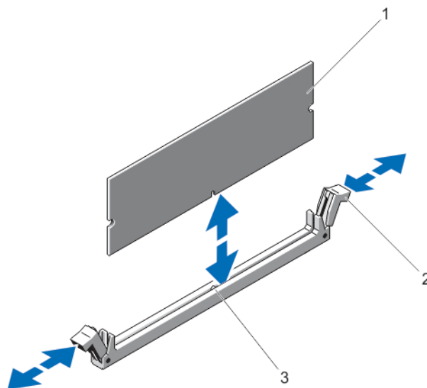
Ilustración 13. Extracción e instalación de un módulo de memoria
