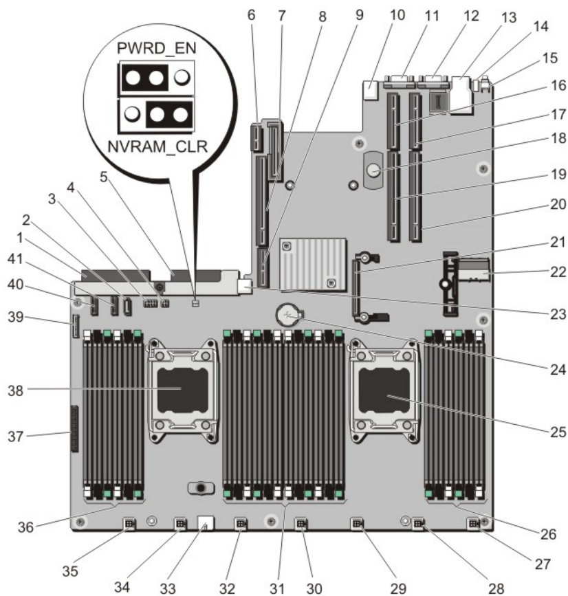
Ilustración 42. Conectores y puentes de la placa base
