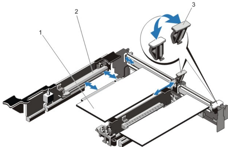
Ilustración 20. Extracción e instalación de la tarjeta de expansión
