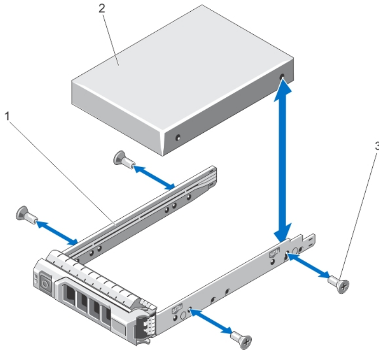
Ilustración 16. Extracción e instalación de una unidad de disco duro en un portaunidades de disco duro
