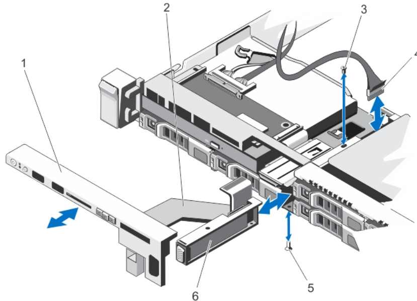
Ilustración 40. Extracción e instalación del módulo VGA
