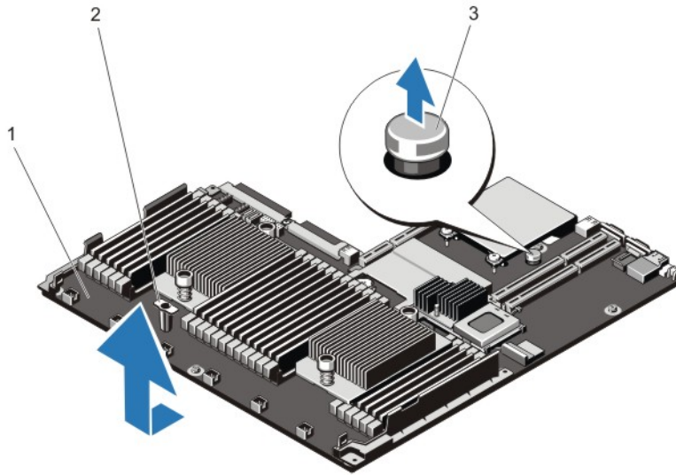
Ilustración 41. Extracción e instalación de la placa base
