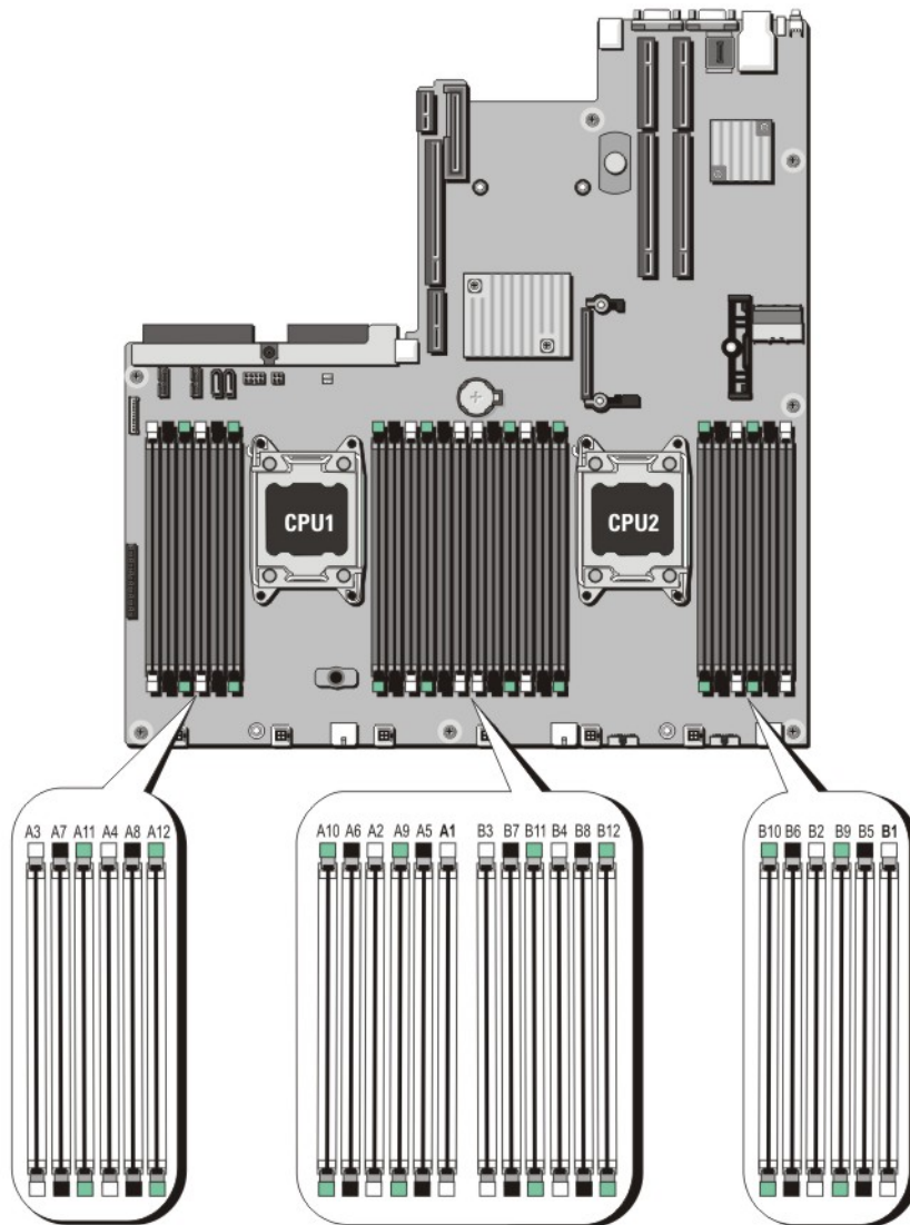
Ilustración 12. Localización de los zócalos de memoria
