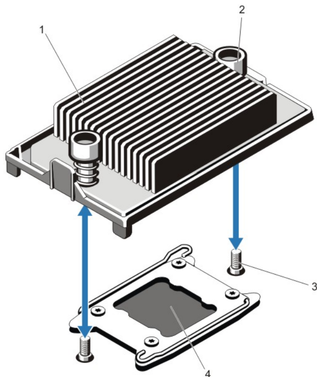
Ilustración 26. Extracción e instalación del disipador de calor
