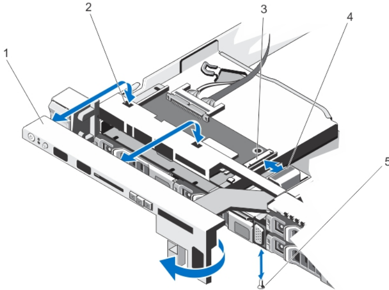
Ilustración 39. Extracción e instalación del panel de control
