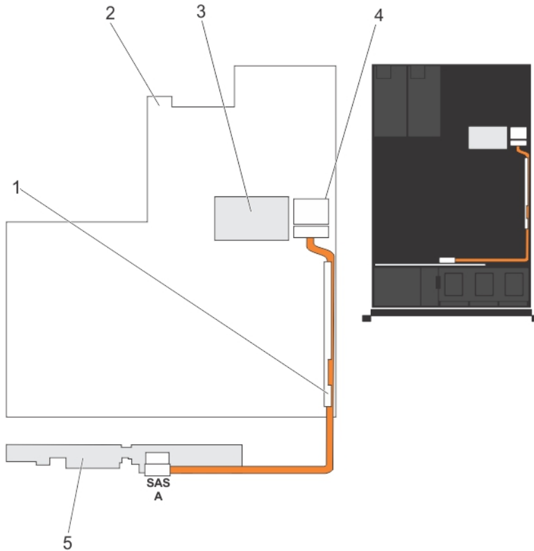
Ilustración 37. diagrama de conexión de cables: sistemas (x4) de 6,35 cm (2,5 pulgadas)
