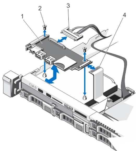
Ilustración 38. Extracción e instalación de la placa del panel de control
