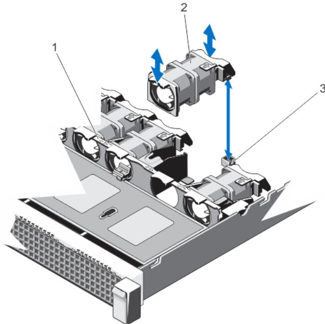
Ilustración 18. Extracción e instalación de un ventilador de enfriamiento
