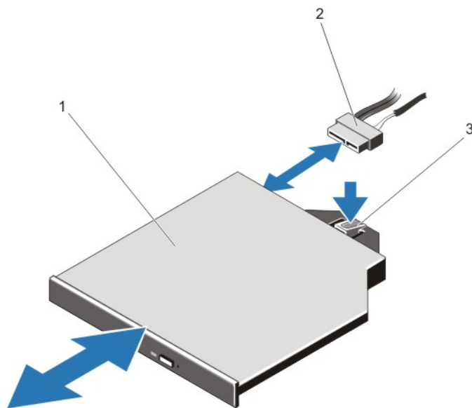
Ilustración 17. Extracción e instalación de la unidad óptica
