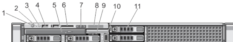
Ilustración 1. Características e indicadores del panel frontal
