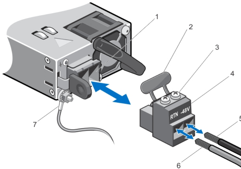
Ilustración 31. Ensamblaje de los cables de alimentación de entrada de CC
